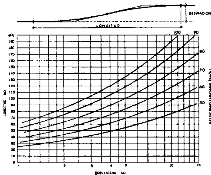
Fig. 34 - LONGITUD MÍNIMA PARA DESVIO PARALELO DE UN CARRIL
