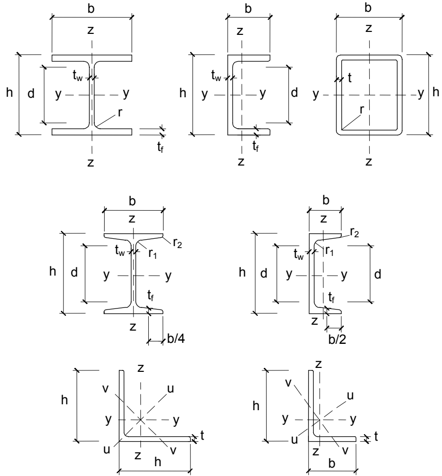
Figura B.1 Dimensiones y ejes de las secciones
