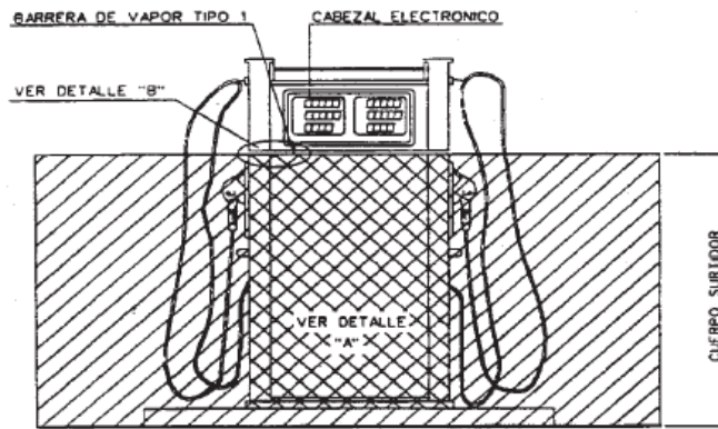
ALZADO
