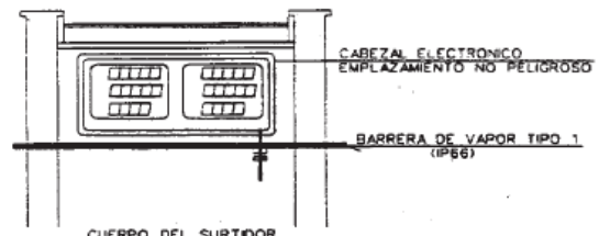
DETALLE "B"
