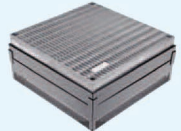
Rejilla para terraza TR-H 40 x 40-95 con pieza de elevación y con tapa elevada
