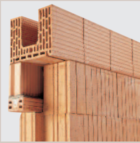
Linteau pour volet roulant monobloc et avec brique Feuillure 12.
