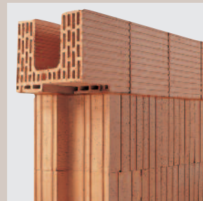
Linteau avec brique Feuillure 12.
