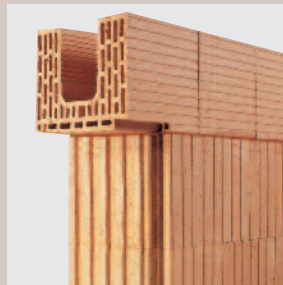
Linteau avec menuiserie au nu intérieur.
