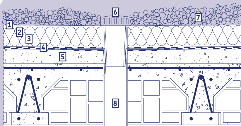
Instalación de sumidero
