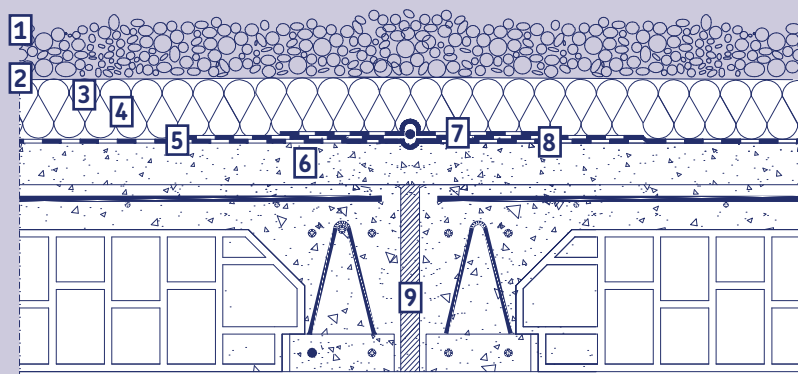
Resolución de junta de dilatación
