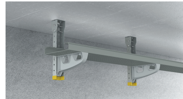
Perfil U perforado metálico disponible en: · Acero inox. AISI 304 con pintura epoxy gris. · Acero galvanizado con pintura epoxy gris. Con soportes horizontales aislantes en U48X.
