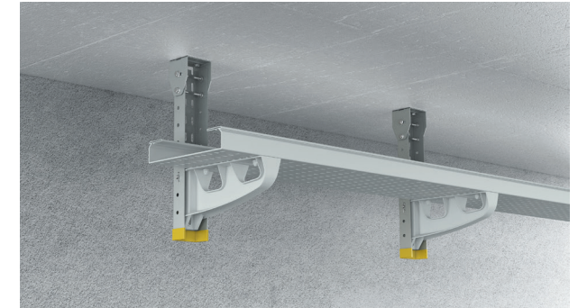
Perfil U perforado metálico disponible en: · Acero inox. AISI 304 con pintura epoxy gris. · Acero galvanizado con pintura epoxy gris. Con soportes horizontales aislantes en U23X y U48X .
