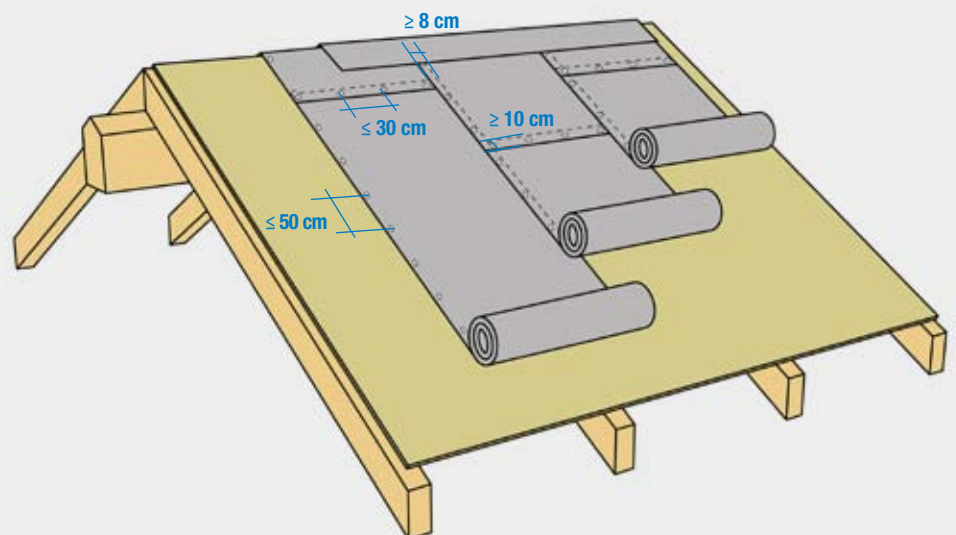
Fig 4.3.6. Fijación mecánica de laminas en pendientes mayores a 50%
