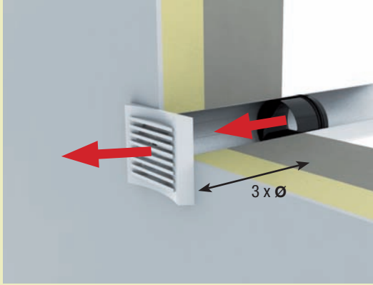
Regulador MRR en insufación
