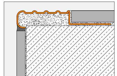
Variante de la instalación Schlüter®-TREP-E
