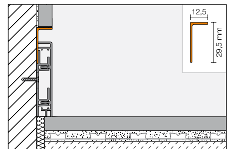
Perfil angular para crear una junta de separación Schlüter®-DESIGNBASE-CQ/SG
