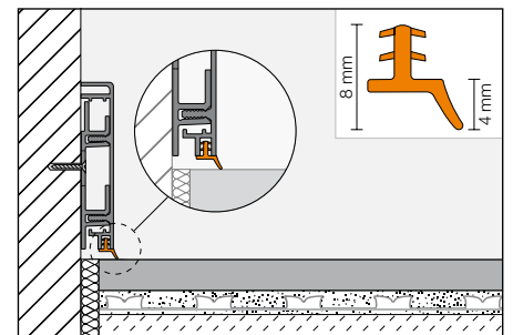
Junta de sellado Schlüter®-DESIGNBASE-CQ/Z
