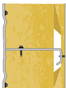
[1] Puente térmico con otra solución estándar.
