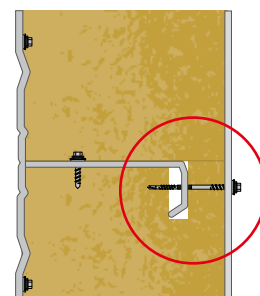
[2] Ausencia de puente térmico con Rockbardage.
