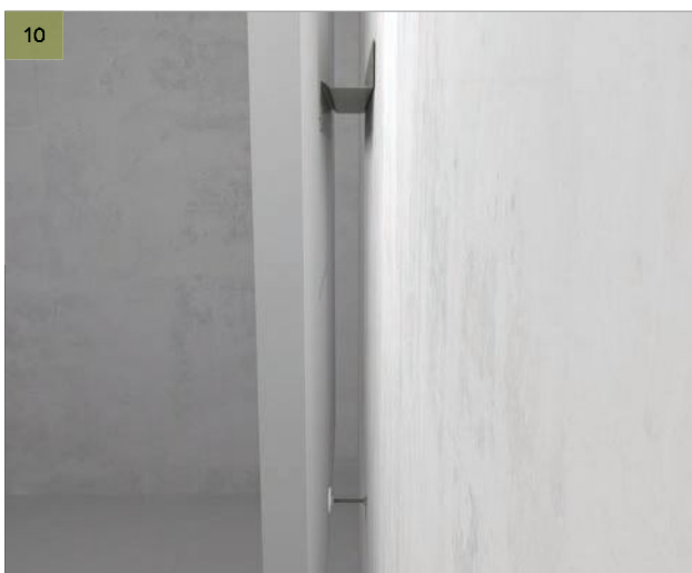
10 Coloque el absorbente mural Rockfon Eclipse en el soporte de fijación en la pared y ajuste el espaciador hasta que el absorbente mural Rockfon Eclipse esté nivelado.
