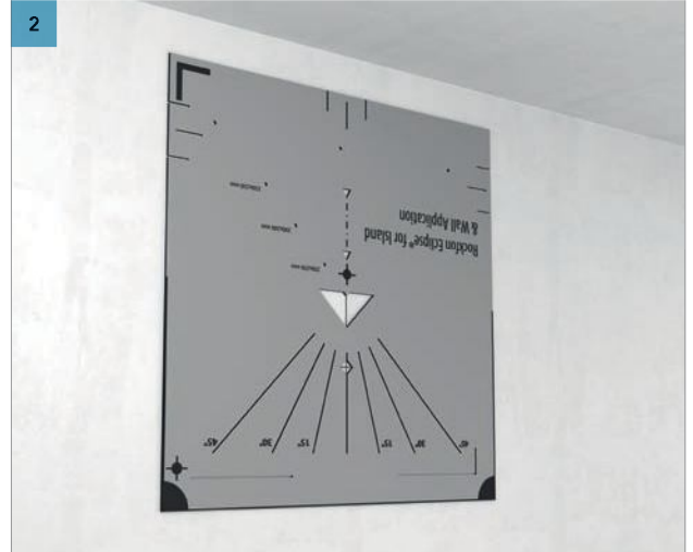
2 Coloque la plantilla sobre las cruces dibujadas en cada lado del punto central del paso 1. Asegúrese de que el centro de la cruz esté alineado con el centro del recorte en forma de rombo de la plantilla. Vea 2 - Detalle
