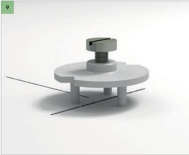
Inserte el espaciador en la parte trasera del absorbente mural. Vea 9 - resultado
