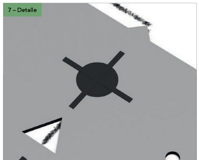
El punto en la base del triángulo debe colocarse en el punto medio de su marcado. La línea que marca el ángulo debe estar alineada con la línea de 0° de la plantilla
