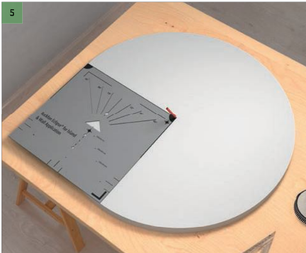
Coloque la plantilla de manera que las esquinas superior izquierda e inferior derecha estén en el borde del círculo en la parte trasera del absorbente mural Rockfon Eclipse. Con un lápiz, marque las líneas centrales utilizando esquinas superior derecha de la plantilla. Vea 5 - Resultado
