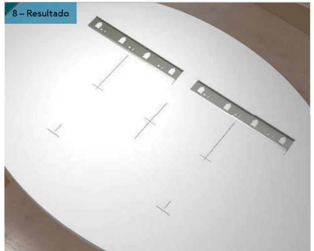
Introduzca el perfil de fijación del panel en el absorbente mural. Vea 8 - Resultado
