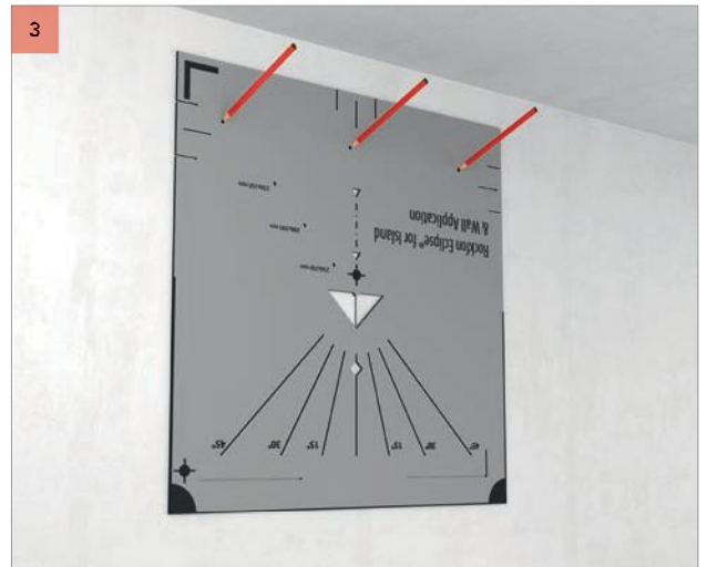
3 Marque puntos para la perforación.
