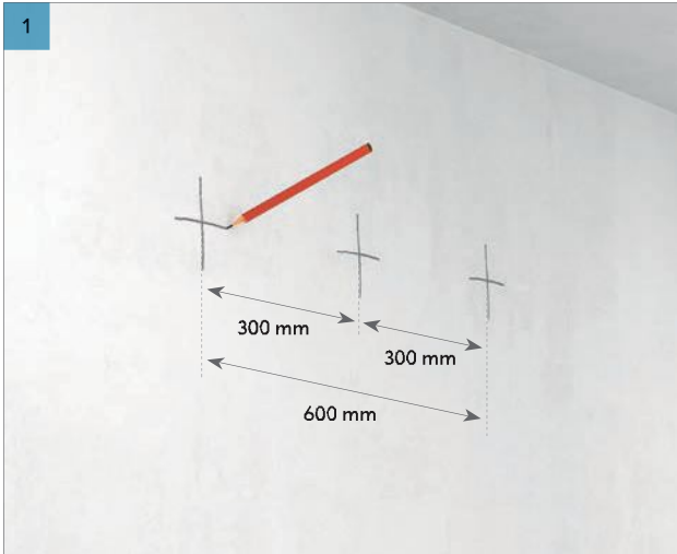
1 Marque cruces en la pared para indicar donde está previsto fijar el absorbente mural Rockfon Eclipse. Dibuje una cruz a 300 mm de cada lado del punto céntrico de la fijación. Asegúrese de que los trazos superiores de las cruces sean de +/- 30 cm
