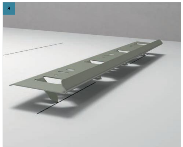
Introduzca el perfil de fijación del panel en el absorbente mural. Vea 8 - Resultado
