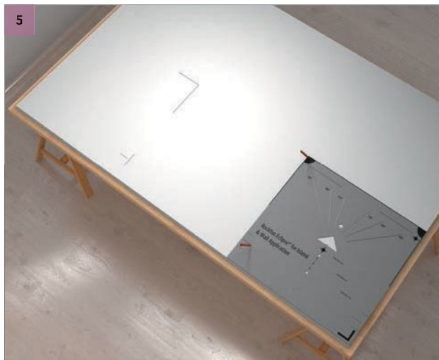
Coloque la plantilla en la esquina inferior derecha de la parte trasera del absorbente mural Rockfon Eclipse. Con un lápiz, marque las líneas centrales, utilizando la esquina superior izquierda de la plantilla y la posición del espaciador. Vea 5 - Resultado.
