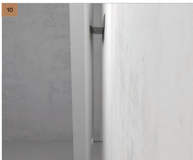
Coloque su absorbente mural Rockfon Eclipse en el perfil de fijación de la pared y ajuste el espaciador hasta que el panel de pared Rockfon Eclipse esté nivelado
