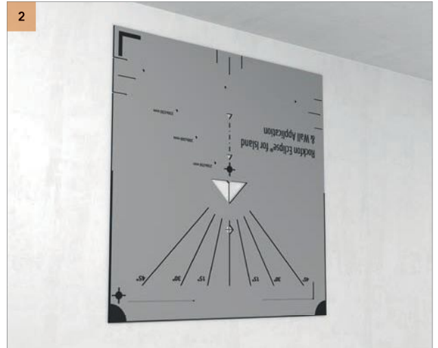
2 Coloque la plantilla sobre la cruz dibujada en el paso 1. Asegúrese de que el centro de la cruz esté alineado con el centro del recorte en forma de rombo de la plantilla. Vea 2 - Detalle
