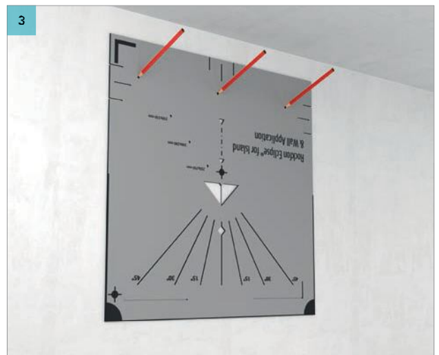
3 Marque puntos para la perforación.
