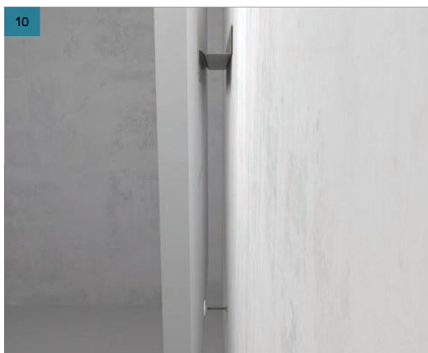
10 Coloque su absorbente mural Rockfon Eclipse en el perfil de fijación de la pared y ajuste el espaciador hasta que el panel de pared Rockfon Eclipse esté nivelado. Vea 10 - Detalle
