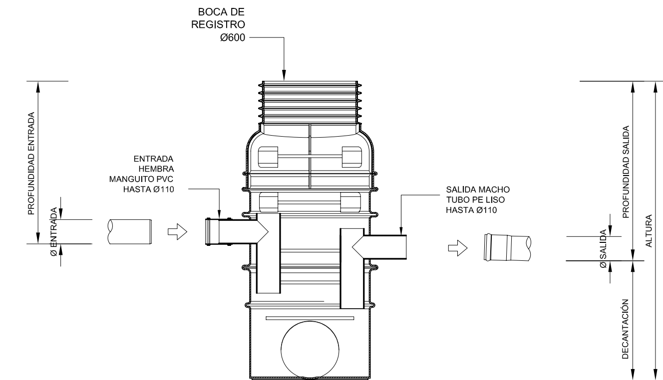
SECCIÓN 1-1
