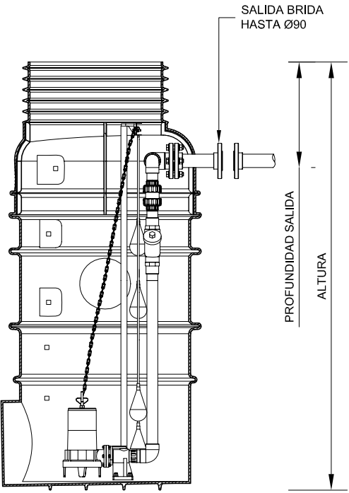
SECCIÓN 2-2
