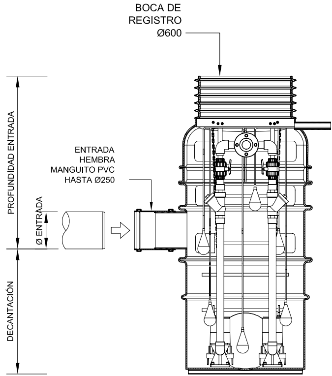
SECCIÓN 1-1
