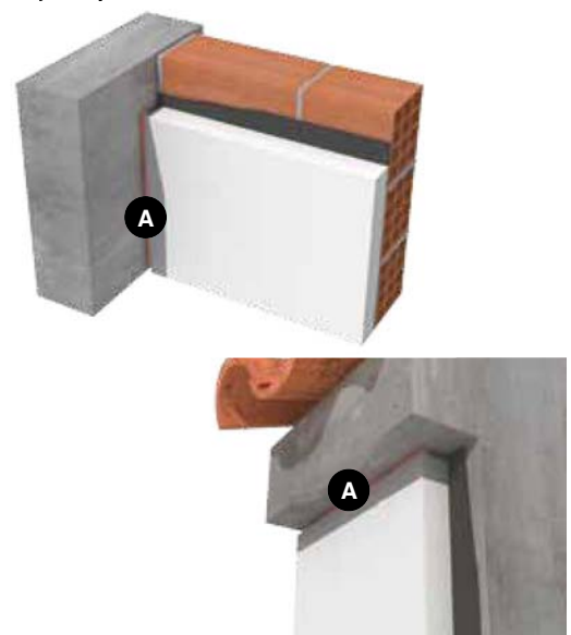
Detalles de aplicación fondo de junta + Pumalastic MS (A)
