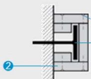
Detalles para fijación a una, dos y tres caras
