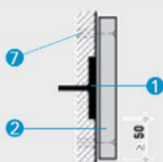
Protección de perfiles tubulares
