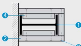
Detalles para fijación a una, dos y tres caras
