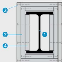
Protección con doble placa
