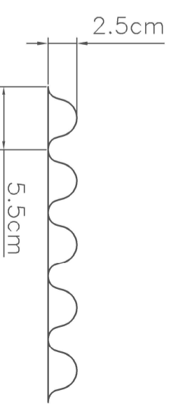
ALZADO DE LA GEOMALLA TRINTER
