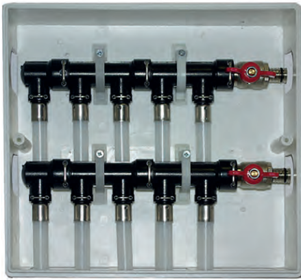
FONTANERÍA / PLUMBING
