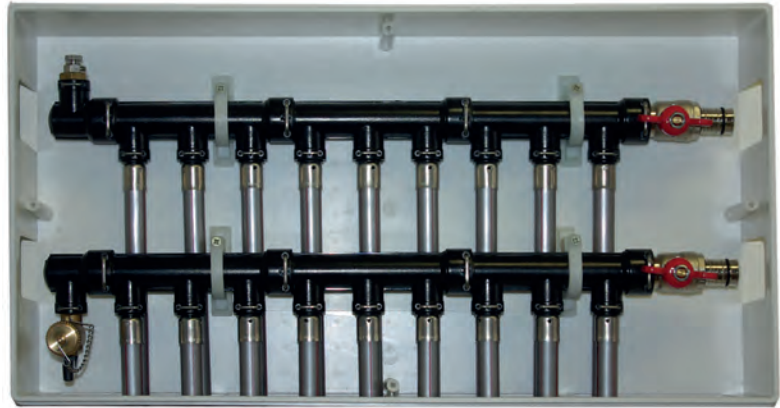
RADIADORES / RADIATORS
