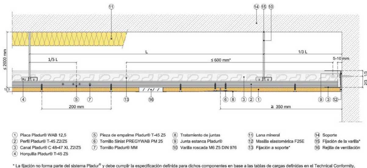
Ilustración 1. Sección longitudinal de techo Pladur® WAB con soporte perimetral resistente y perfil T-45 apoyado en canal perimetral.
