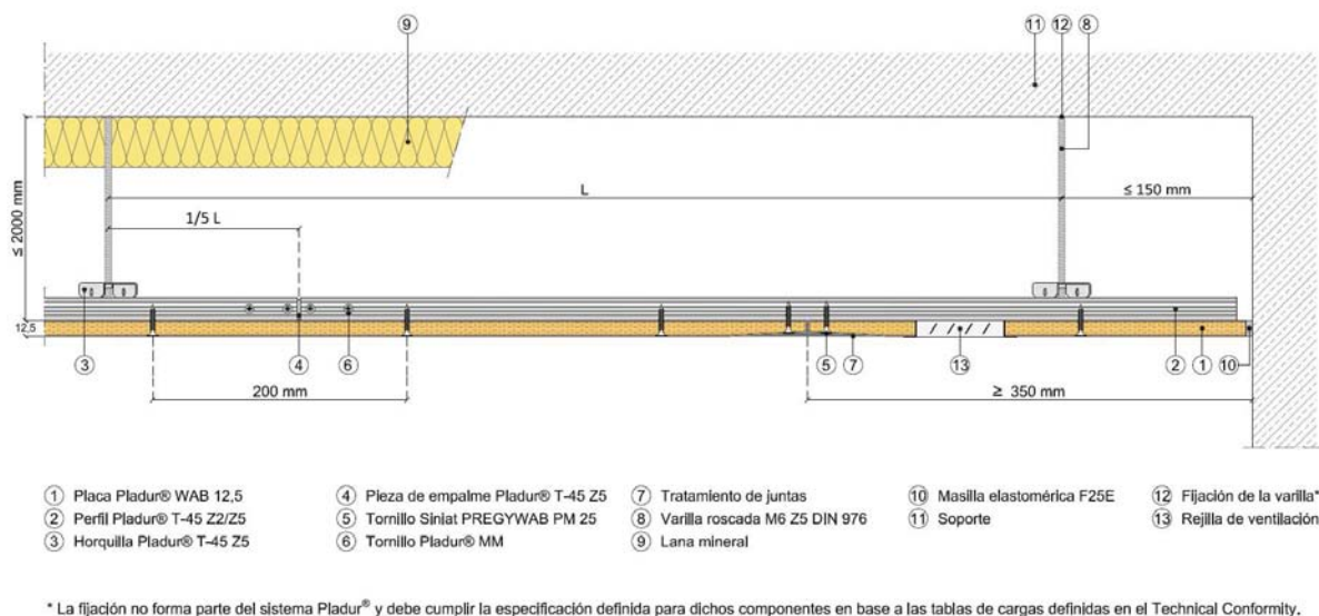
Ilustración 2. Sección longitudinal de techo Pladur® WAB con soporte perimetral no resistente.
