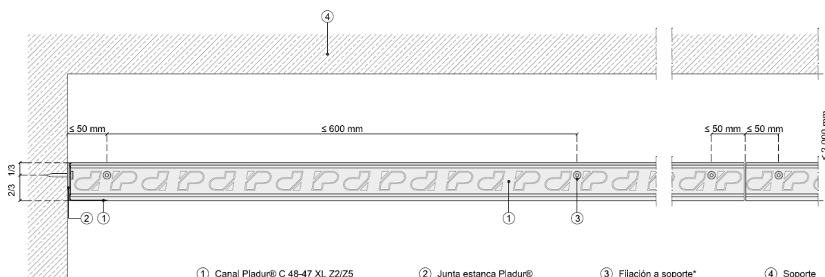
Ilustración 12. Instalación de canal perimetral.
