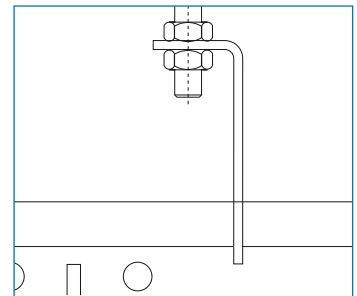
Sección de la pieza de cuelgue
