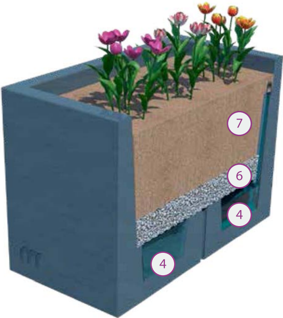
Sección esquemática del sistema de riego eficiente MyR
