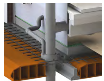
Ejemplo de instalación embutido
