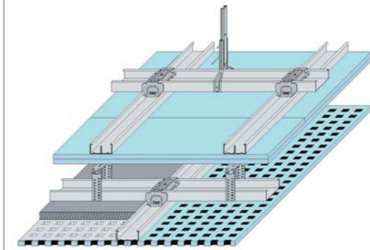
Techo suspendido Knauf D112
