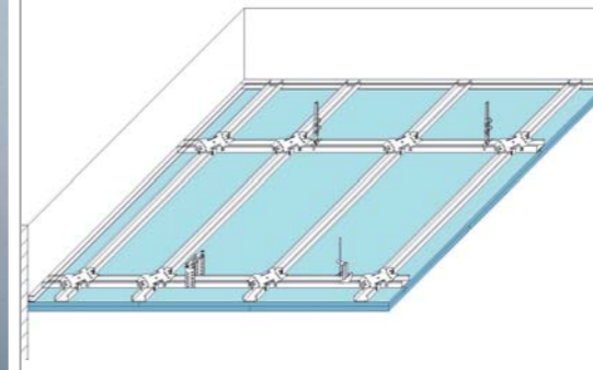
El secreto: empalme en cruz
