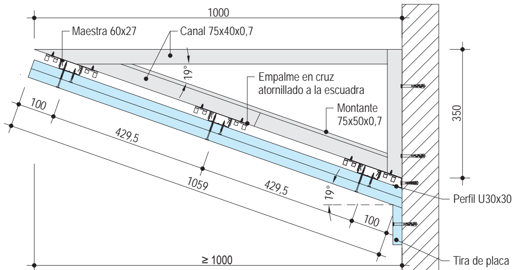
Dimensiones de escuadra metálica.
