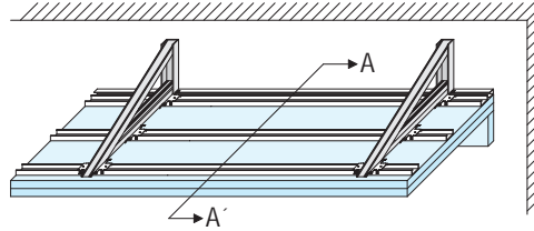
Perspectiva Isométrica
