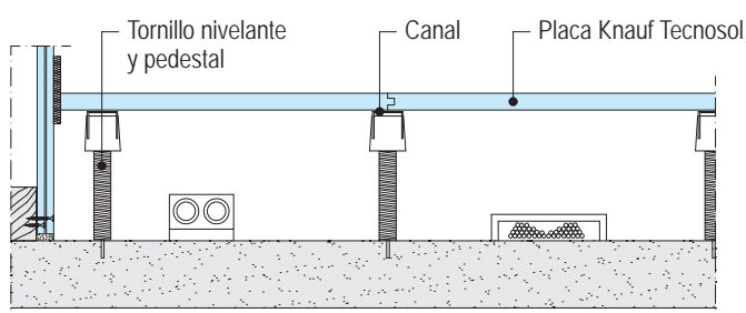
F191.es-V18 Suelo Técnico Tecnosol sobre apoyos Sistema Granab 7000 (Esc. 1:12,5)
