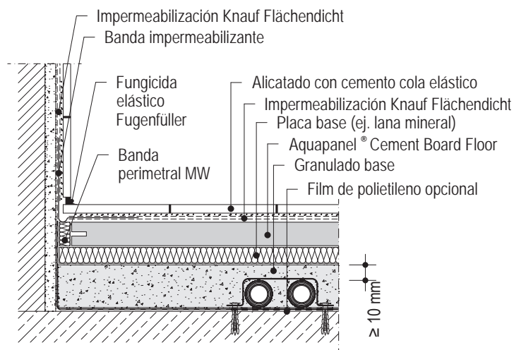
F154.es-V5 Nivelación con granulado base
