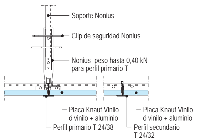
D143.es-A4 Encuentro entre primario y secundario
