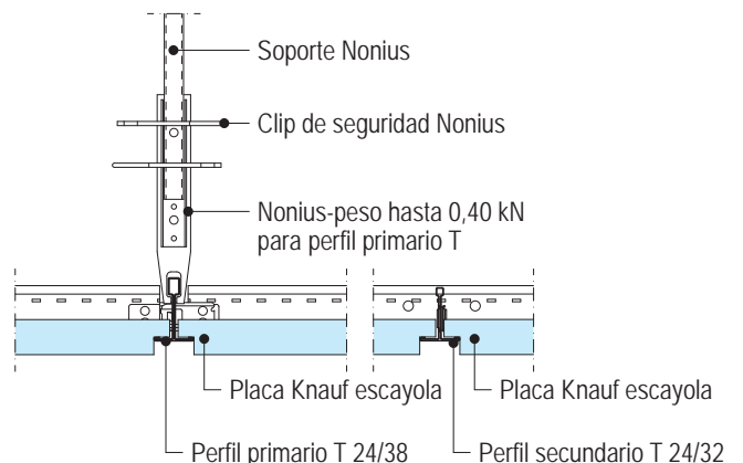
D142b.es-A2 Encuentro entre primario y secundario
