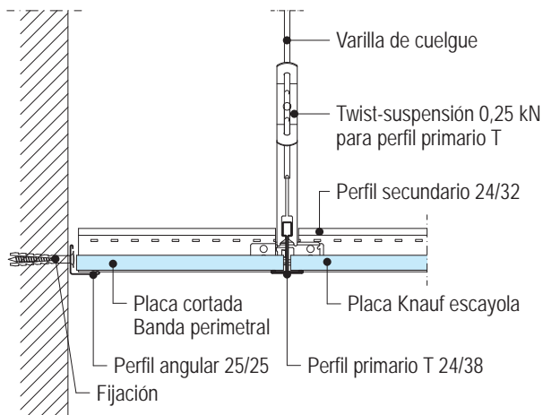
D142b.es-A1 Banda perimetral con angular transversal al perfil primario
