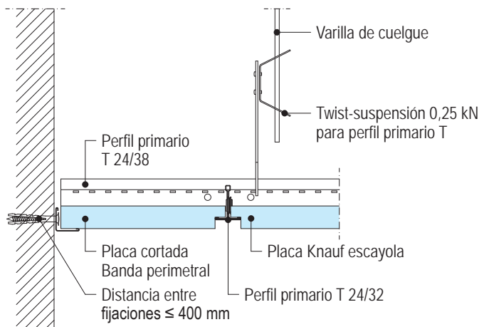
D142b.es-A1 Banda perimetral con angular transversal al perfil primario
