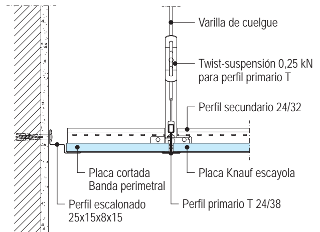
D142b.es-A2 Encuentro entre primario y secundario
