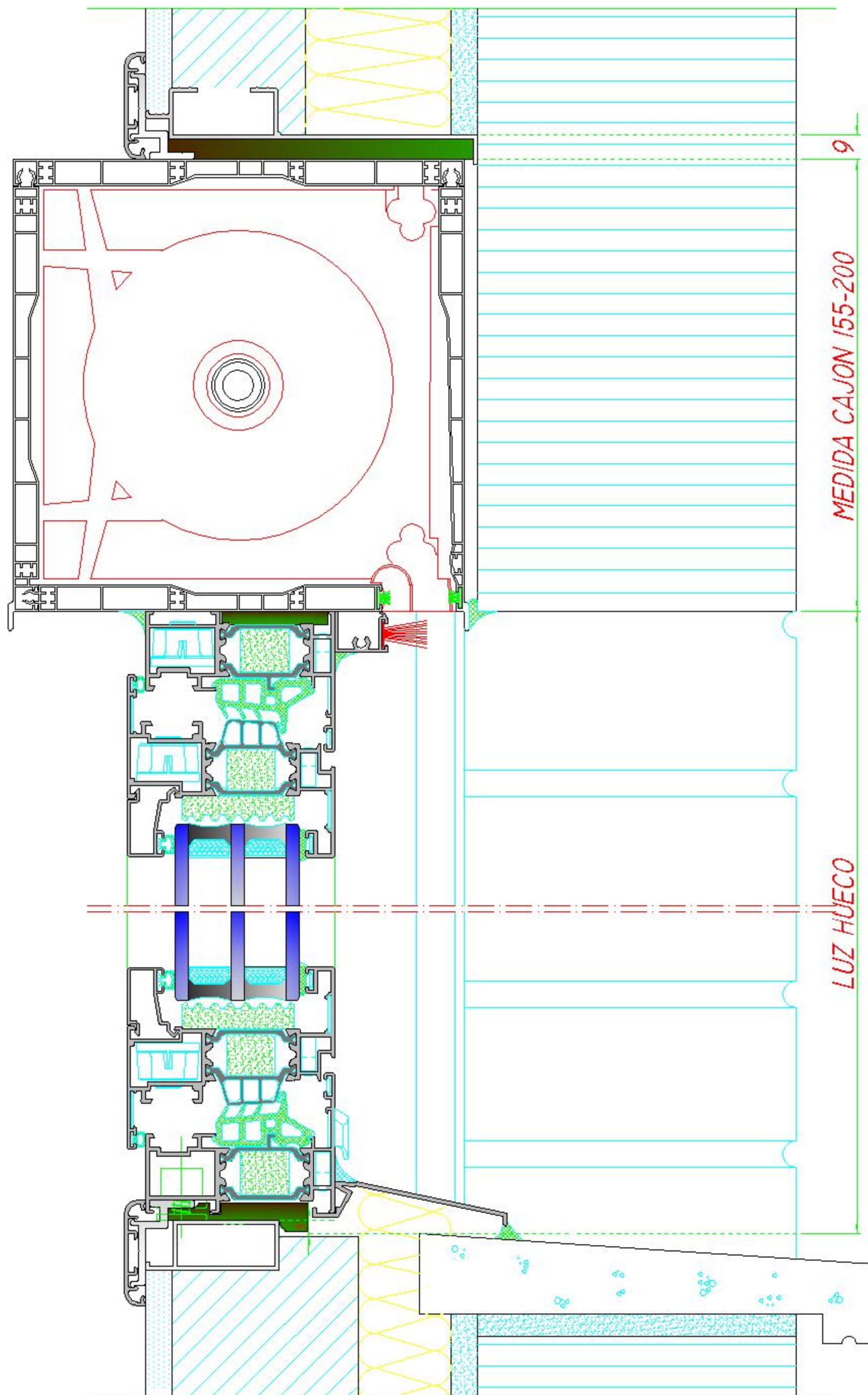
SECCION VERTICAL 71RPT INSTALACION PERSIANA CON GUIAS
