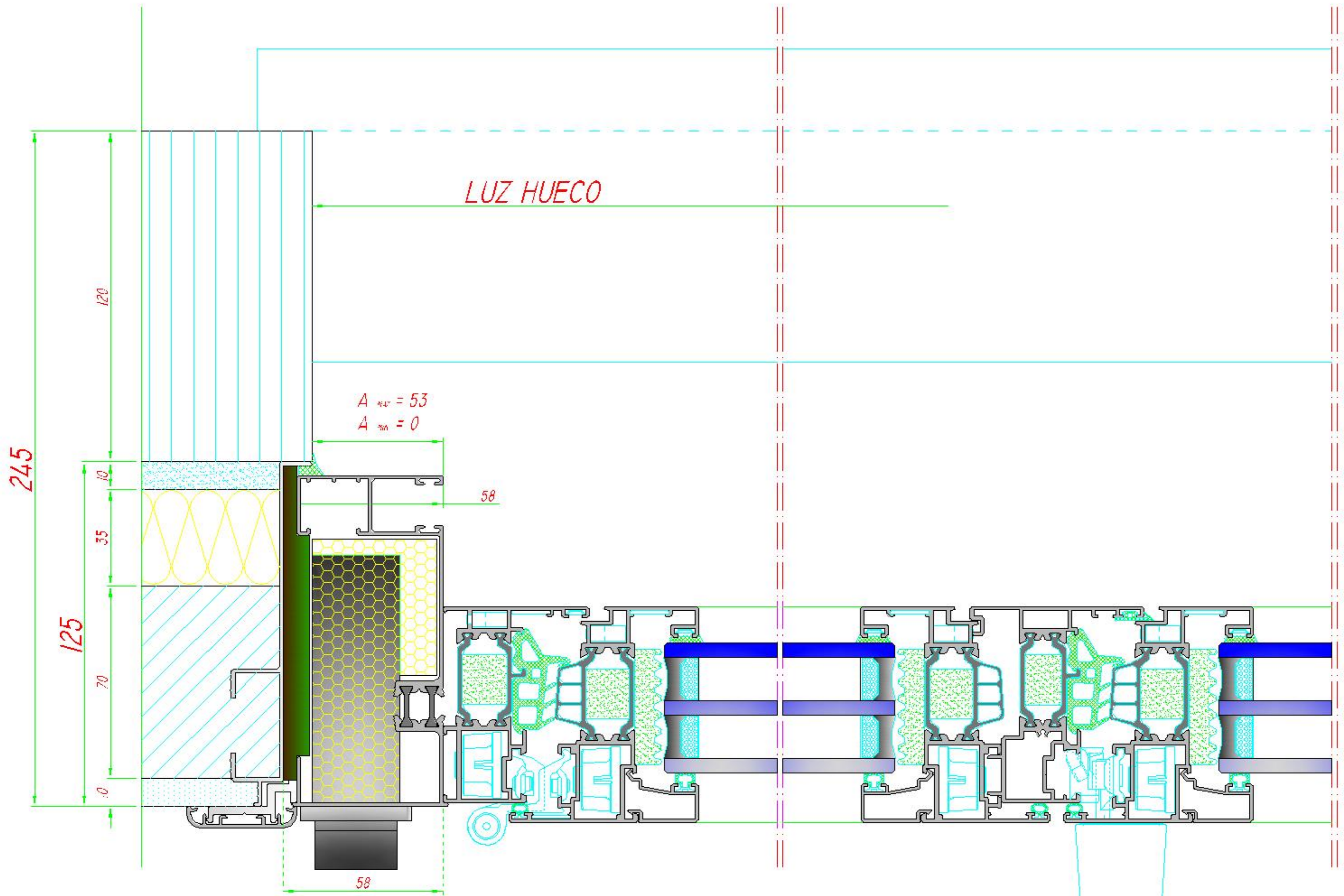
SECCION HORIZONTAL 71RPT INSTALACION PERSIANA CON GUIA
