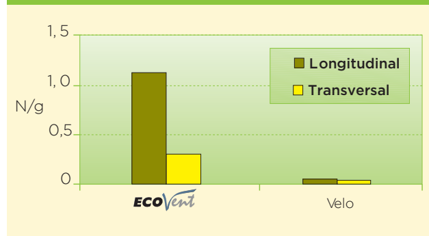
Comparativa de la resistencia mecánica de un revestimiento de tejido neto y un revestimiento velo.
