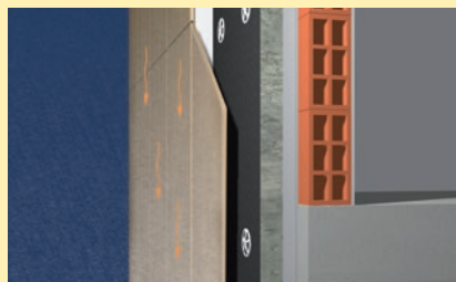
5. La estructura externa de la fachada ventilada aísla el edificio contra las inclemencias externas como el viento o la lluvia.
