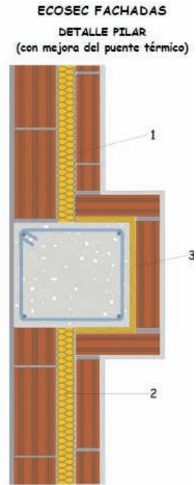
Fig. 4: Detalle de encuentro con pilar
