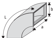
Codo curvo
