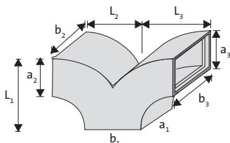
Pantalón curvo
