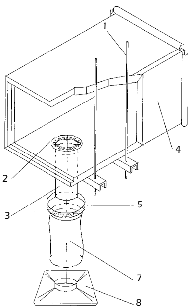
Difusor redondo
