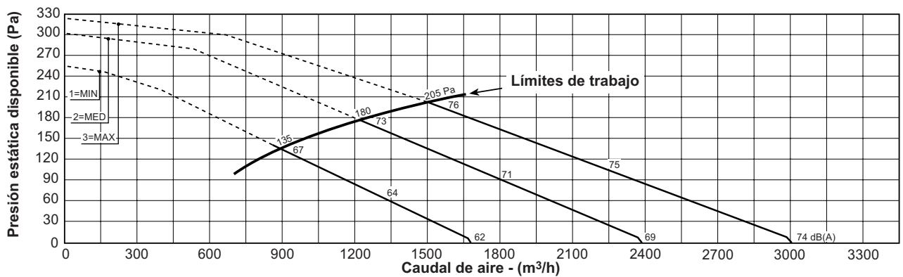
MOD.: BSW 60 - SISTEMA DE 2 TUBOS (datos bobina 4R)
