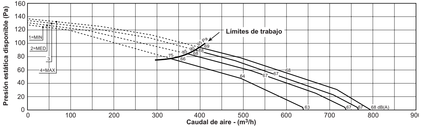
MOD.: BSW 20 - SISTEMA DE 4 TUBOS (datos bobina 3R+1R)
