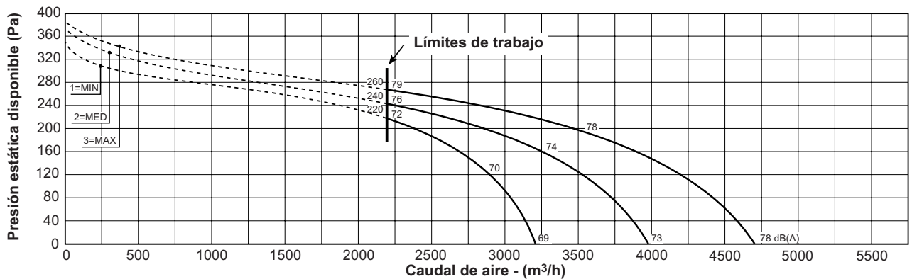
MOD.: BSW 70 - SISTEMA DE 2 TUBOS (datos bobina 4R)
