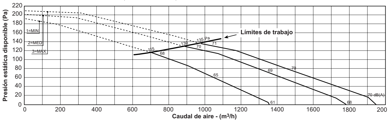
MOD.: BSW 30 - SISTEMA DE 2 TUBOS (datos bobina 3R)
