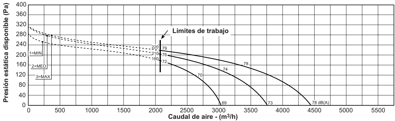
MOD.: BSW 70 - SISTEMA DE 4 TUBOS (datos bobina 4R+2R)
