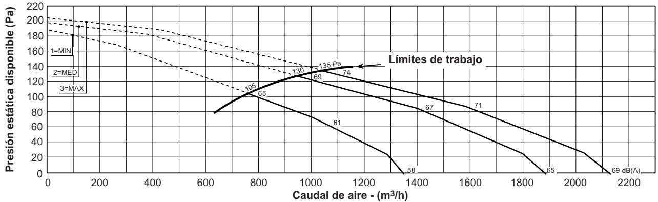
MOD.: BSW 50 - SISTEMA DE 2 TUBOS (datos bobina 3R)
