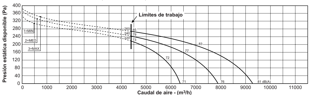
MOD.: BSW 70 - SISTEMA DE 2 TUBOS (datos bobina 4R)
