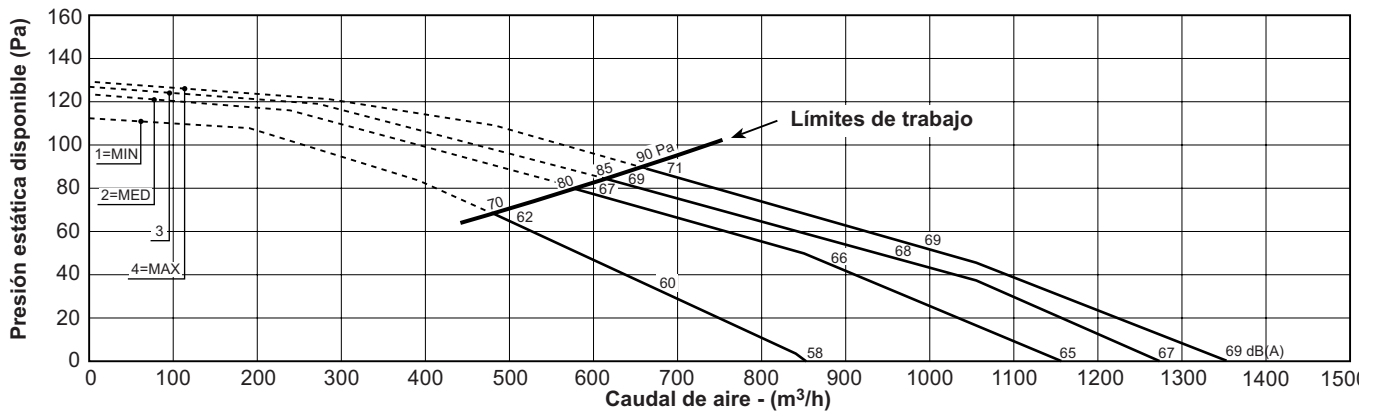
MOD.: BSW 30 - SISTEMA DE 4 TUBOS (datos bobina 3R+1R)
