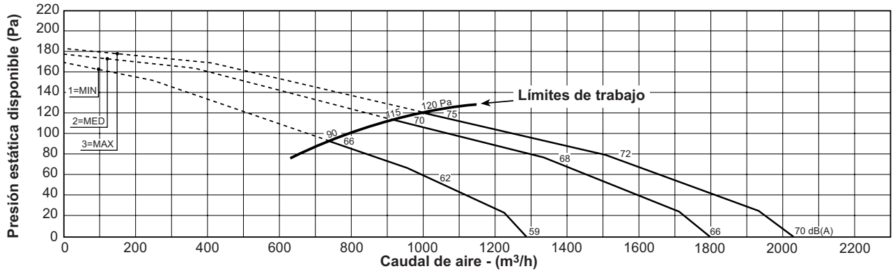
MOD.: BSW 50 - SISTEMA DE 4 TUBOS (datos bobina 3R+1R)
