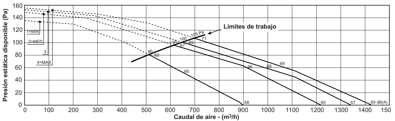
MOD.: BSW 20 – SISTEMA DE 2 TUBOS (datos bobina 3R)
