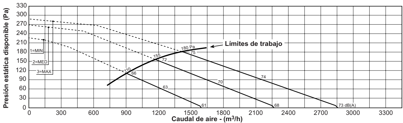
MOD.: BSW 60 - SISTEMA DE 4 TUBOS (datos bobina 4R+2R)
