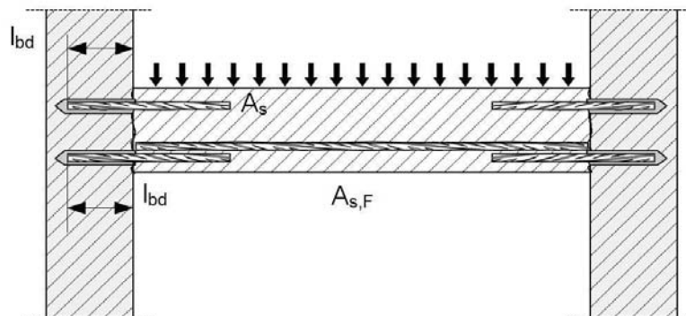
Figure A3 : Ancrage d'armatures en extrémité de dalles ou de poutres
