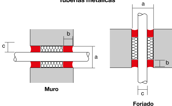
Tuberías metálicas
