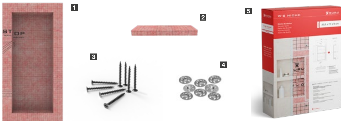
1- Hornacina prefabricada W-S NICHE. 2- Estante. 3- Tornillos (x8). 4- Arandelas metálicas (x8). 5- Caja W-S NICHE.
