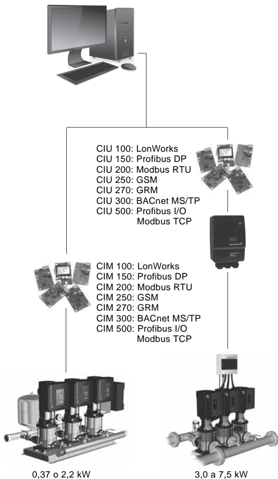
Fig. 13 Estructura del sistema de gestión de edificios
