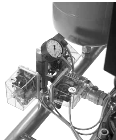
Fig. 22 Interruptores de presión en el colector
