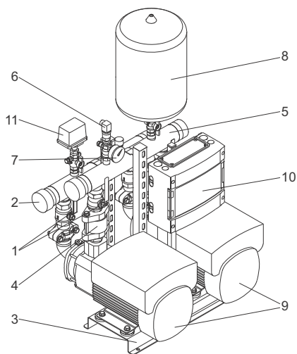
Fig. 5 Hydro Multi-E con dos bombas CME
