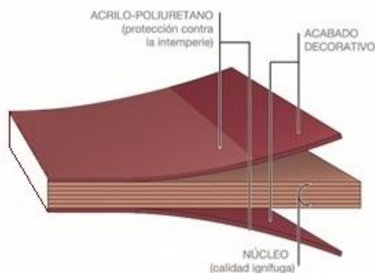
Figura 2.1a: Composición de los paneles Max® Exterior.
