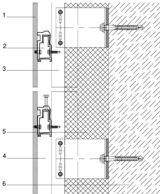
Figura 5.1: Sección vertical.
