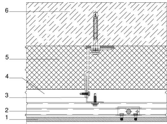
Figura 5.2: Sección horizontal.
