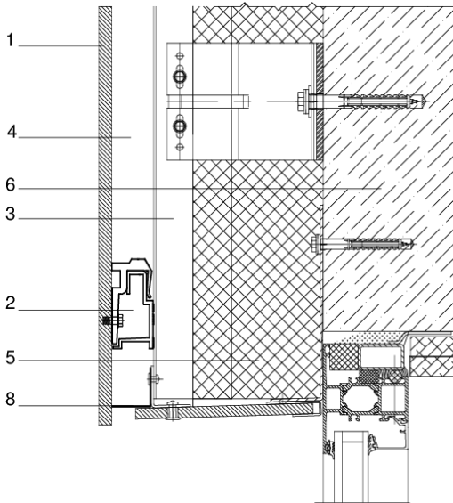
Figura 5.10: Sección vertical. Dintel.
