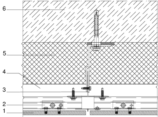
Figura 5.6 Sección horizontal. Continuidad de perfil guía horizontal.
