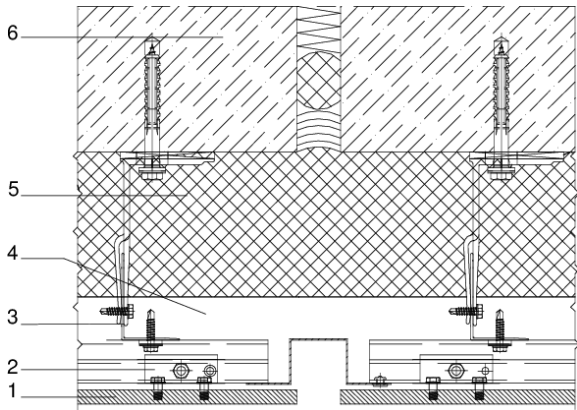
Figura 5.18: Sección horizontal. Junta estructural.
