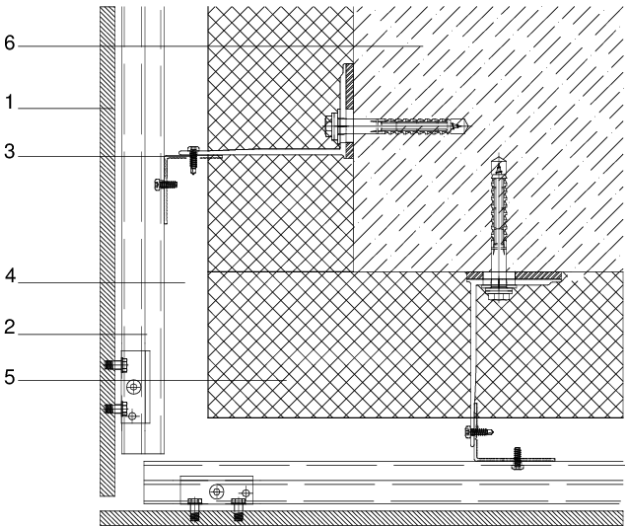
Figura 5.15: Sección horizontal. Esquina saliente.
