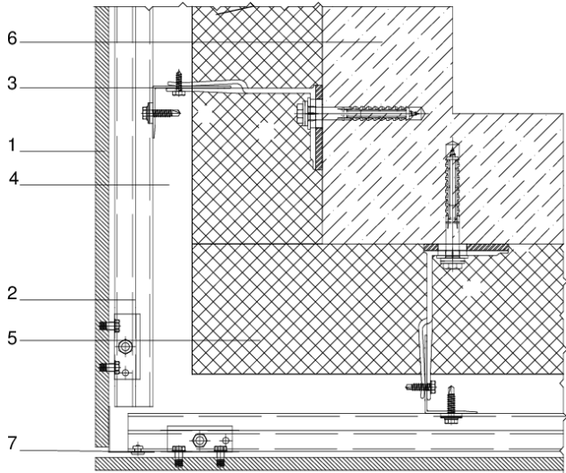
Figura 5.16: Sección horizontal. Esquina saliente con perfil auxiliar.
