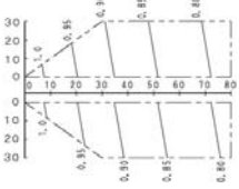
Relación de corrección para capacidad de refrigeración
