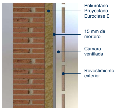
Solución con revestimiento de mortero genérico.
