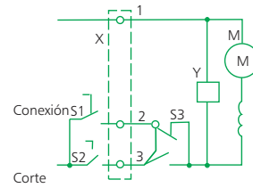
Sin relé de cierre automático
