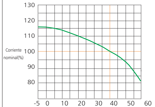
Curva de compensación de temperatura para NM1-63(40~63), NM1-125(40~125)
