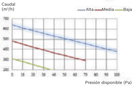
ERV 500-1
