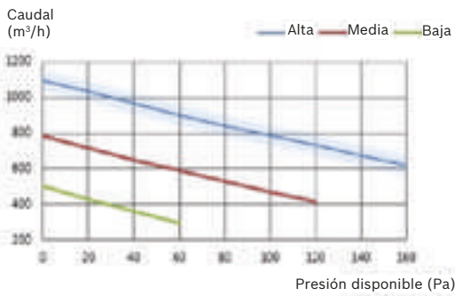
ERV 800-1
