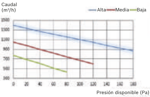
ERV 1000-1
