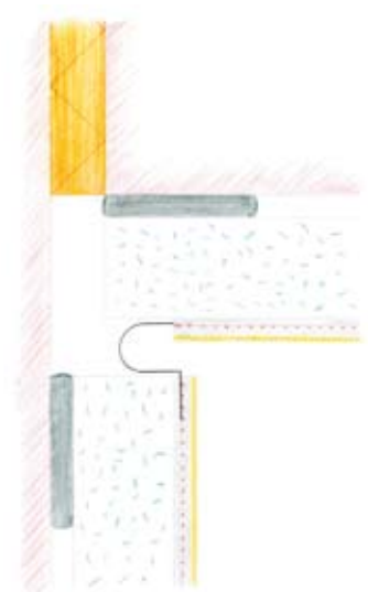
Figura 25 Juntas de compensación en V
