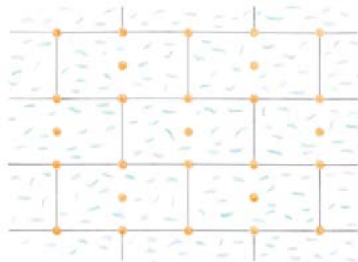
Figura 21 Espigado en T en paneles de material aislante de EPS-F
