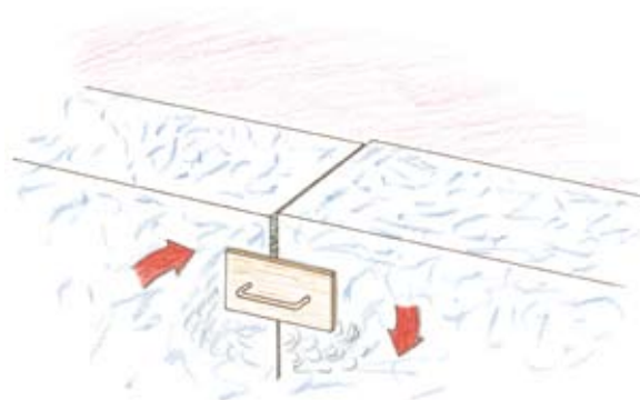
Figura 19 Pulido de las juntas de los paneles aislantes
