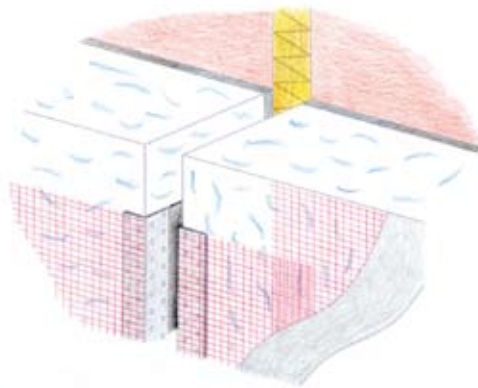
Figura 26 Utilización Baunit DehnfugenProfil en E
