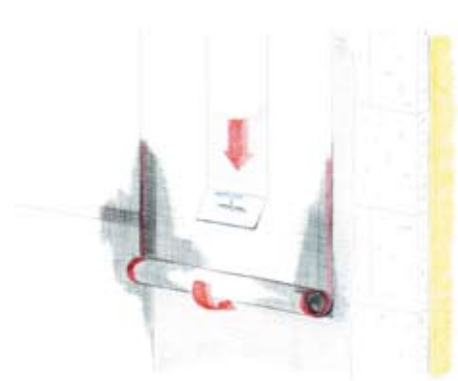
Figura 37 Encastrado de la rejilla Baunit TextilglasGitters "húmedo sobre húmedo"
