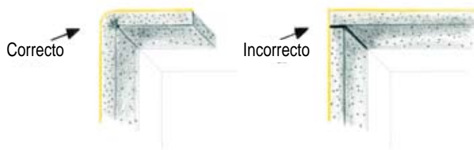
Figura 27 Baunit FugendichtBand unidas a testa
