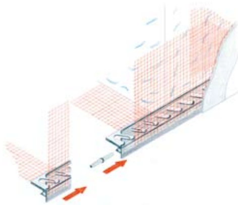
Figura 36 Aplicación Baunit TropfkantenProfil
