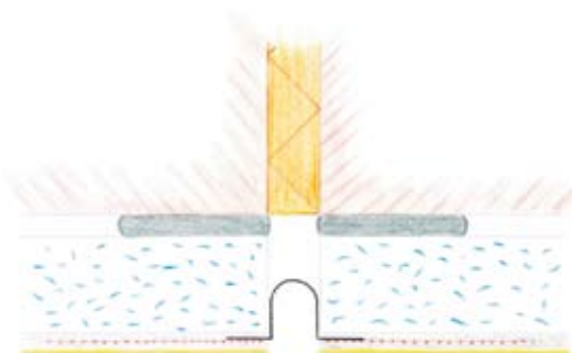
Figura 24 Juntas de compensación en E
