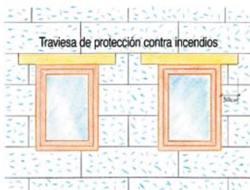
Figura 1 Montaje a la altura del dintel de la ventana
