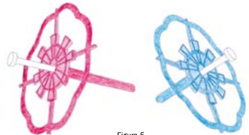
Figura 5 Baumit KlebeAnker (rojo) y Baumit KlebeAnker Betón (azul)
