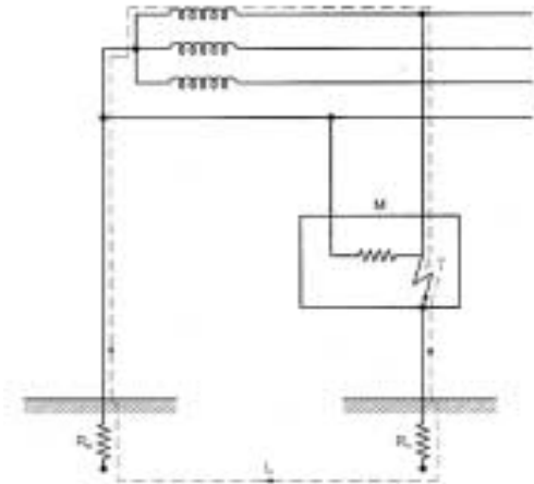
Figura 4 Esquema TT
