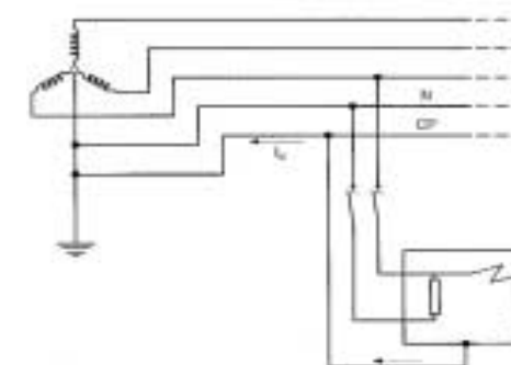
Figura 3. Esquema TN-S.
