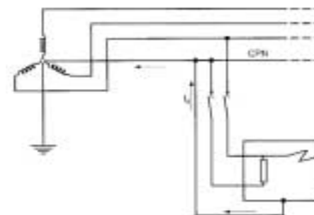
Figura 2. Esquema TN-C.
