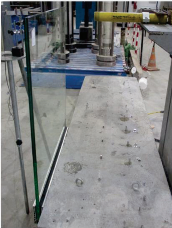
Aspecto tras el empuje horizontal hacia el exterior
